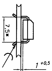
В(3) Установка ДАЗ
