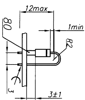
Установка VD3
