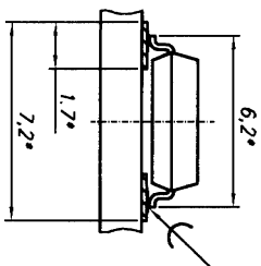
Установка ДА1 5:1
