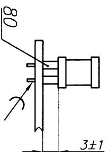
Установка L2
