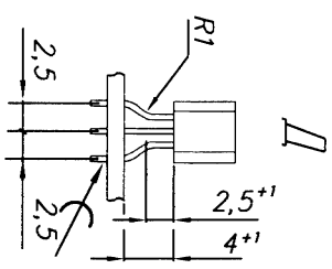
Вариант установки ДАЗ поз.29
