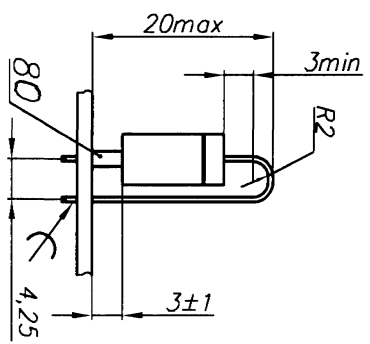
Установка VD2, VD5
