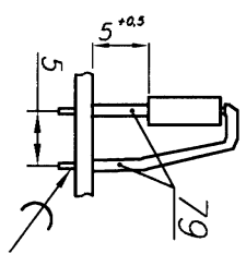
Установка FU1
