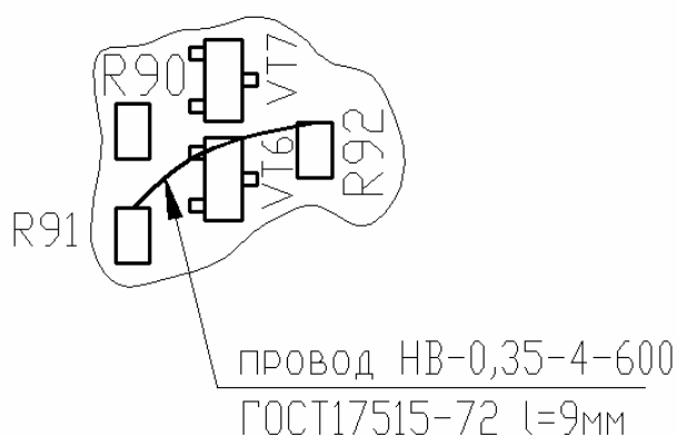
Схема разделки перемычки
